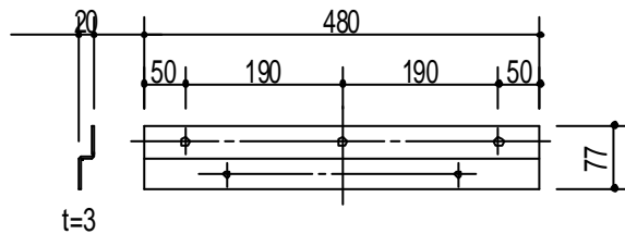
本体取付金具 (2本付)
